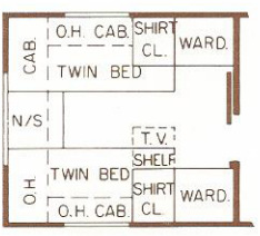
OPT. BEDROOM
