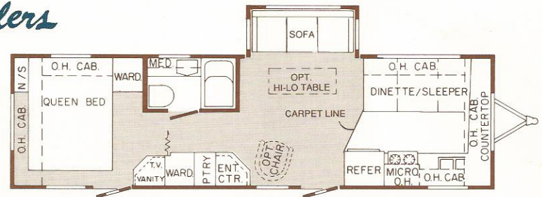
32' DALLAS AXLE WT. 7635 HITCH WT. 850
